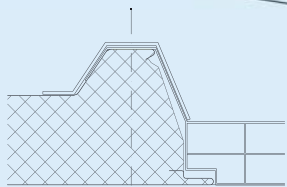
Unterkonstruktion substructure
